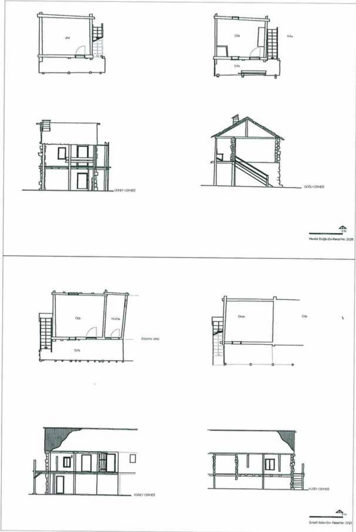
Çizim 1. 215/1 İsmail Aslan ve 215/8, Mevlüt Eroğlu Evi Plan ve Görünüşleri
